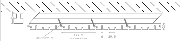
Detail Deckenmontage Querschnitt [M 1:10]
