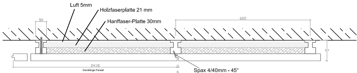
Detail Deckenmontage Längsschnitt [M 1:10]
